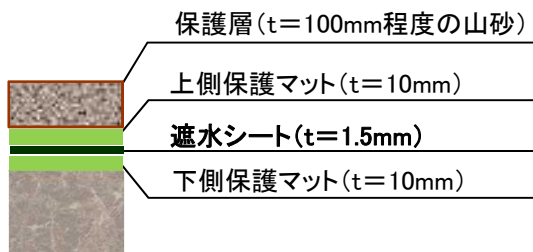
底面部分の詳細構造(例)
