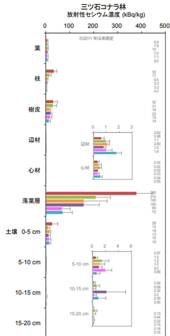
各調査地における部位別放射性セシウム濃度(kBq/kg、平均値)の変化
